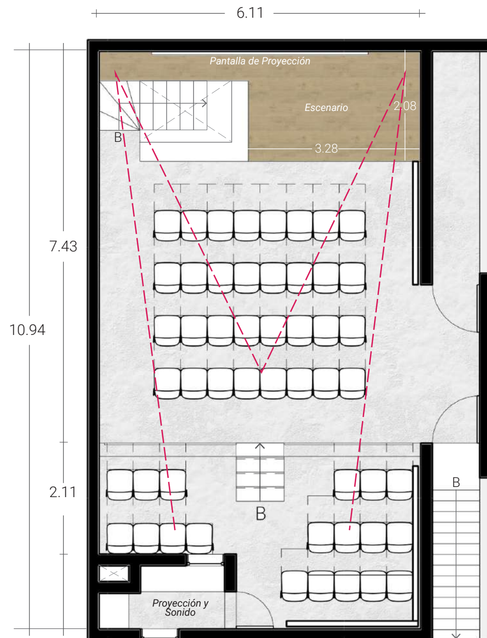
Planta Auditorio
