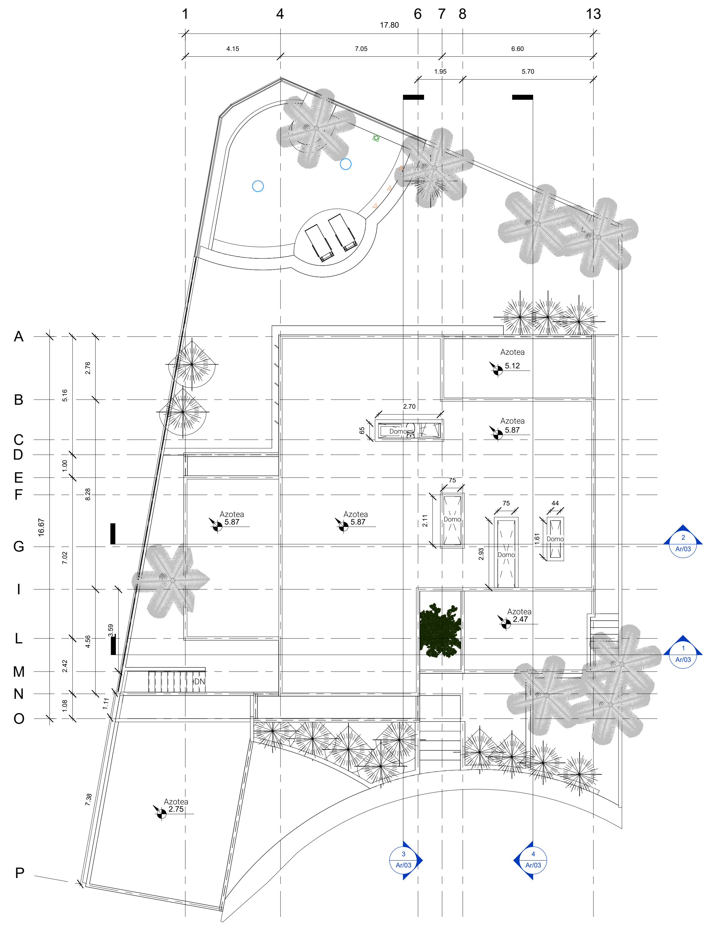
1 Planta Conjunto 1 : 100
