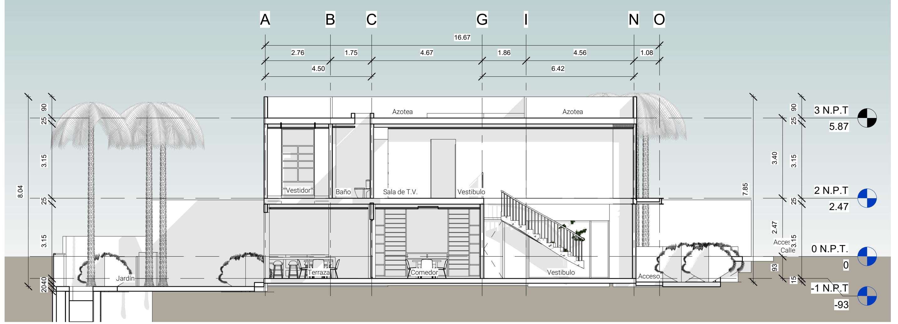
3 Sección 3 1 : 100
