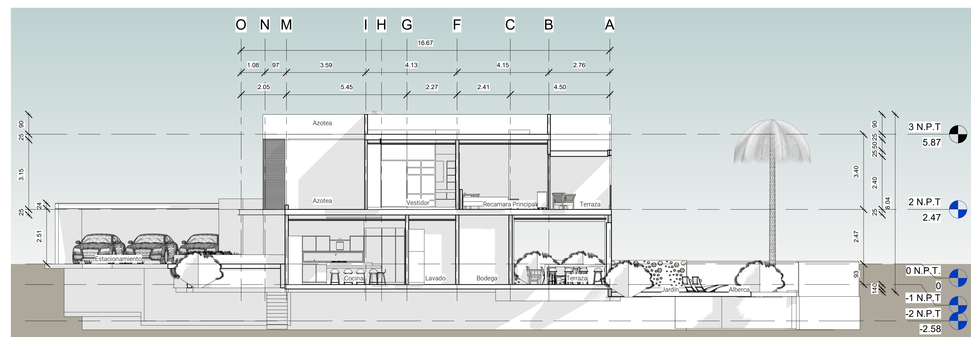
4 Sección 4 1 : 100
