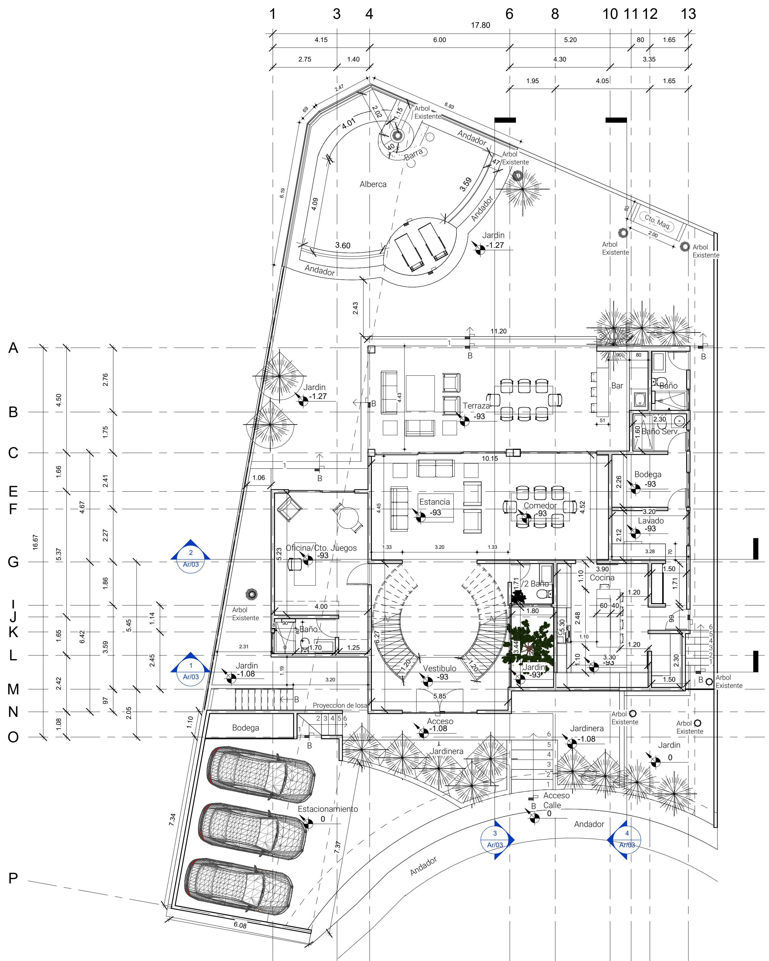
1 Planta Baja 1 : 100
