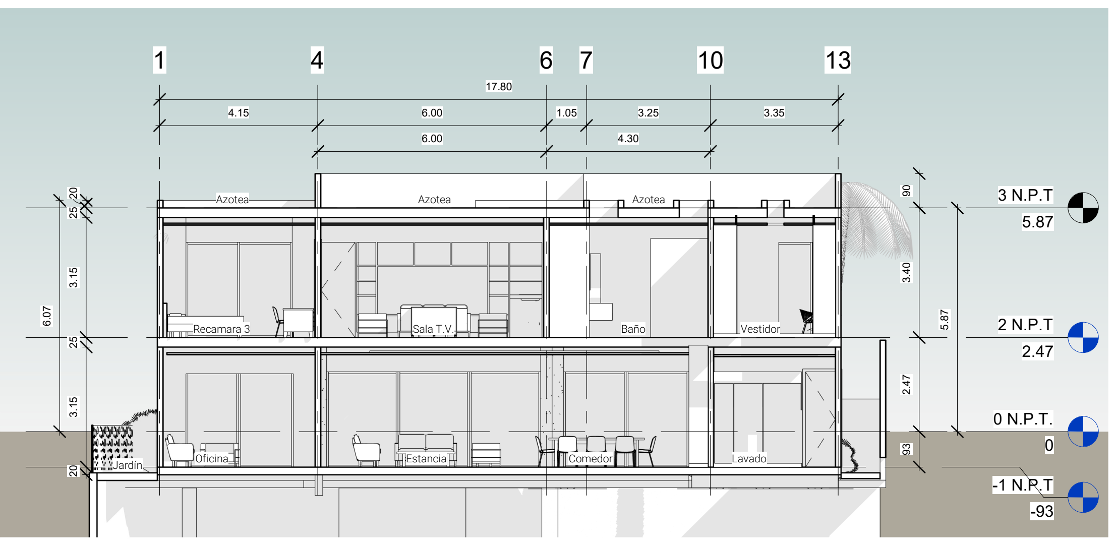
2 Sección 2 1 : 100
