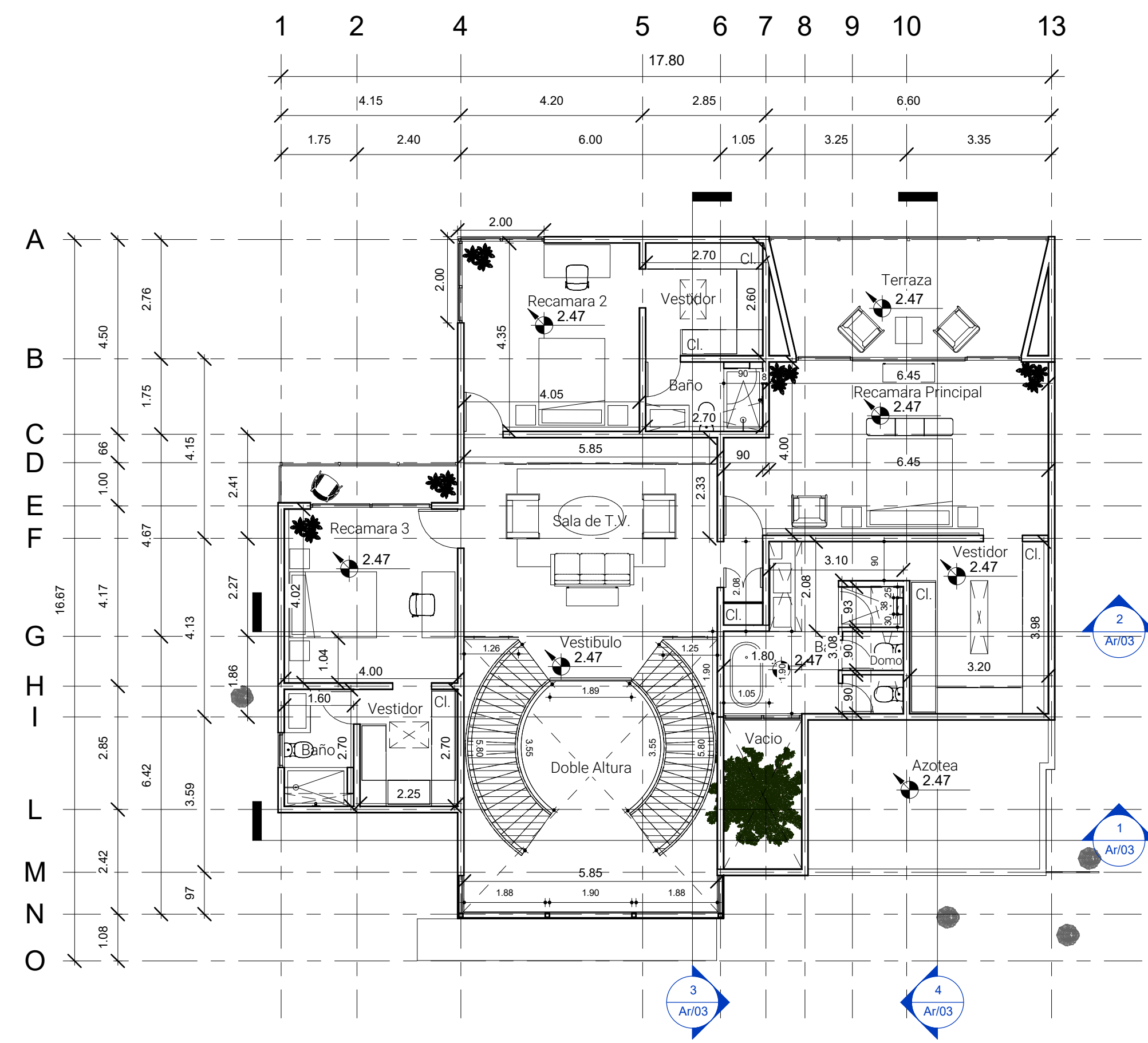
2 Planta Alta 1 : 100
