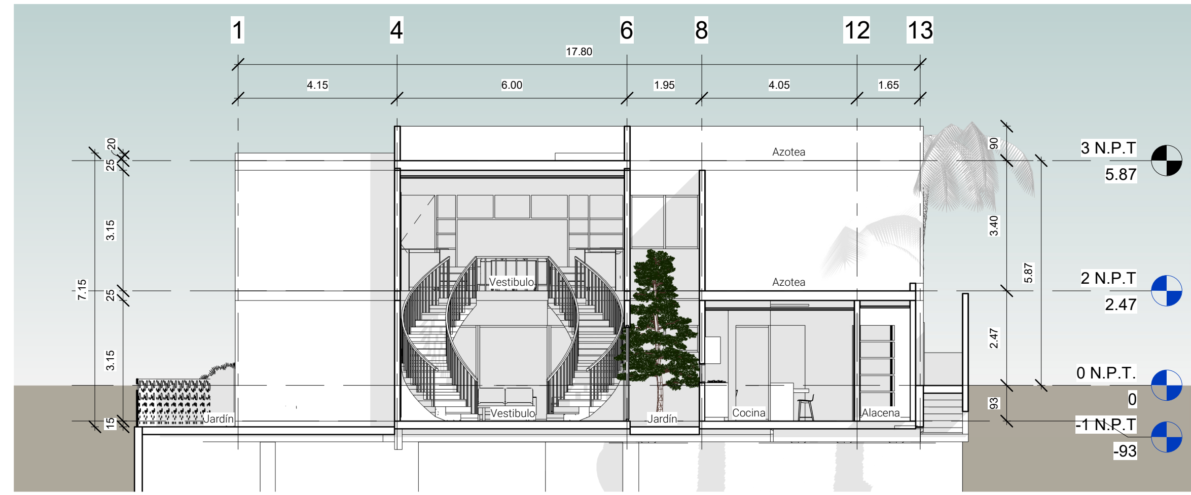
1 Sección 1 1 : 100
