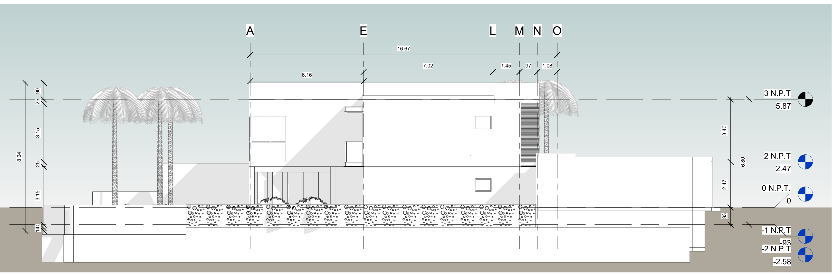
4 Fachada Oeste 1 : 100
