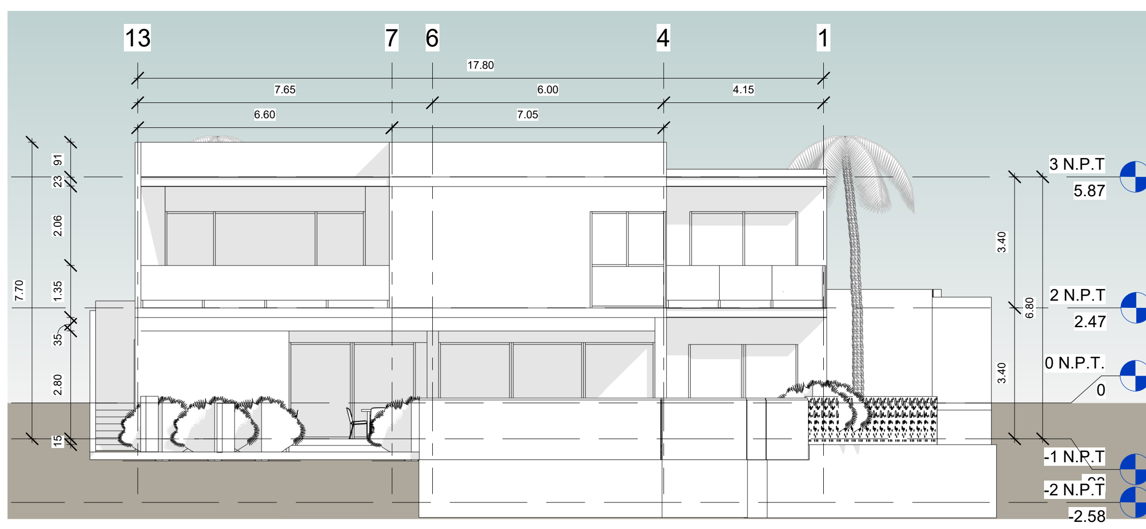
4 Fachada Norte 1 : 100
