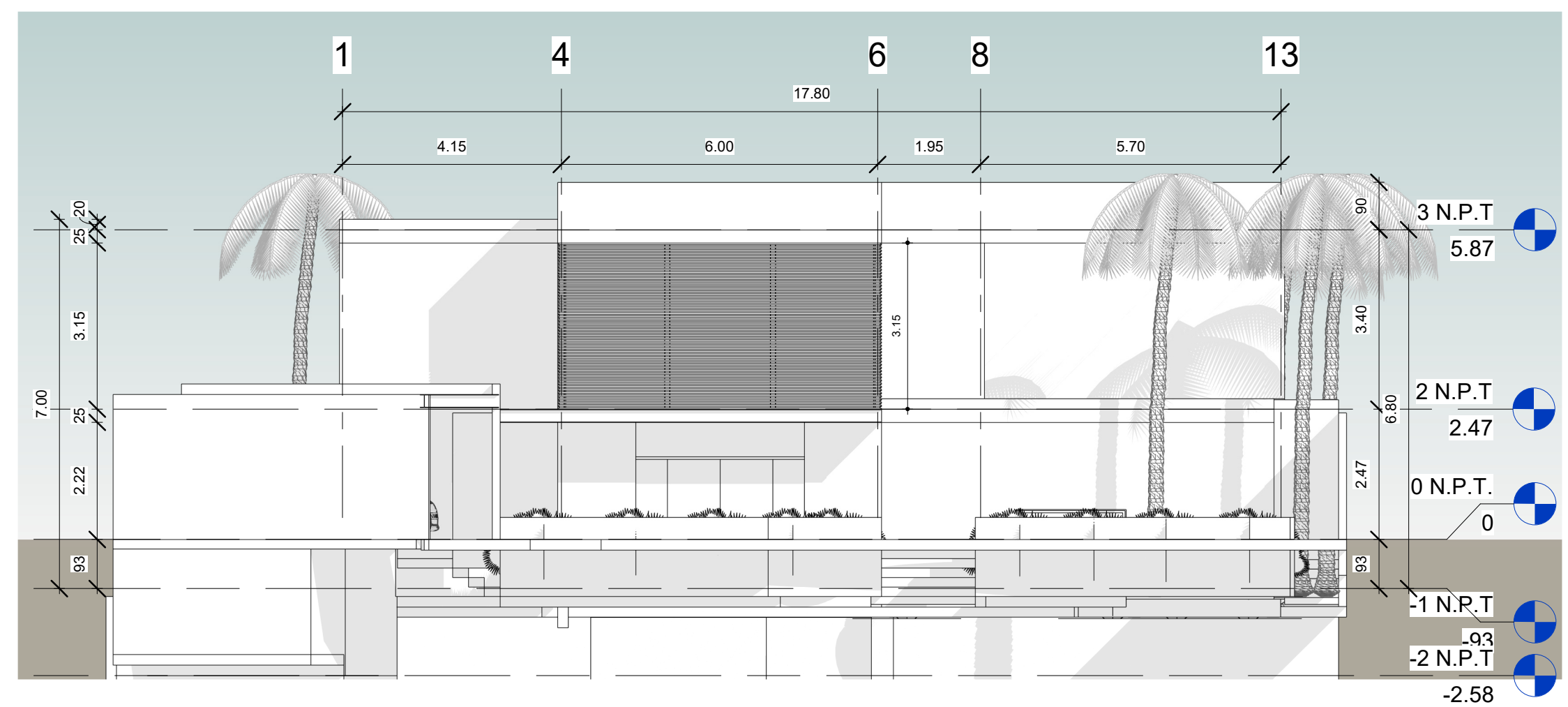
3 Fachada Sur 1 : 100
