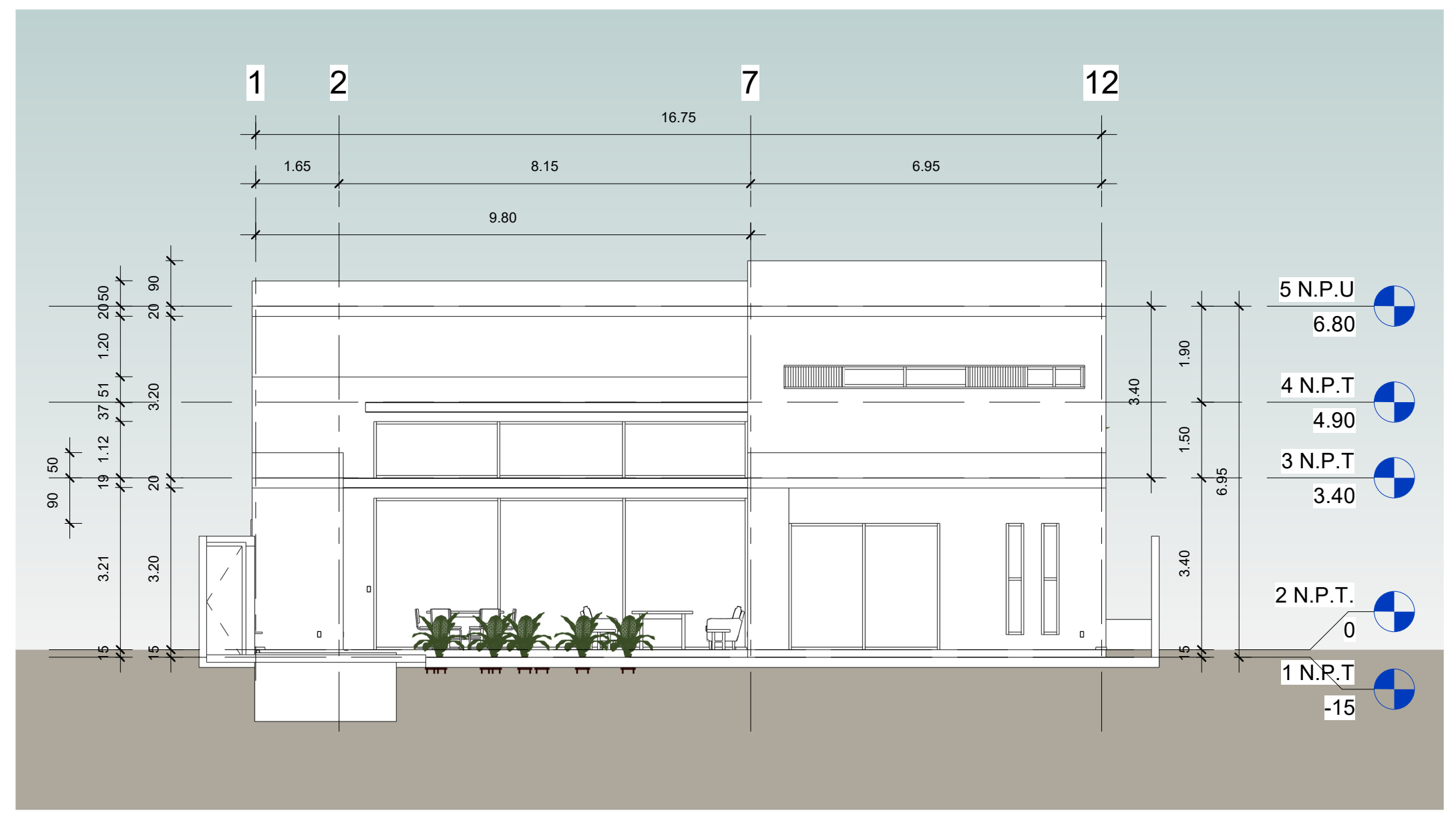
4 Fachada Este 1 : 100
