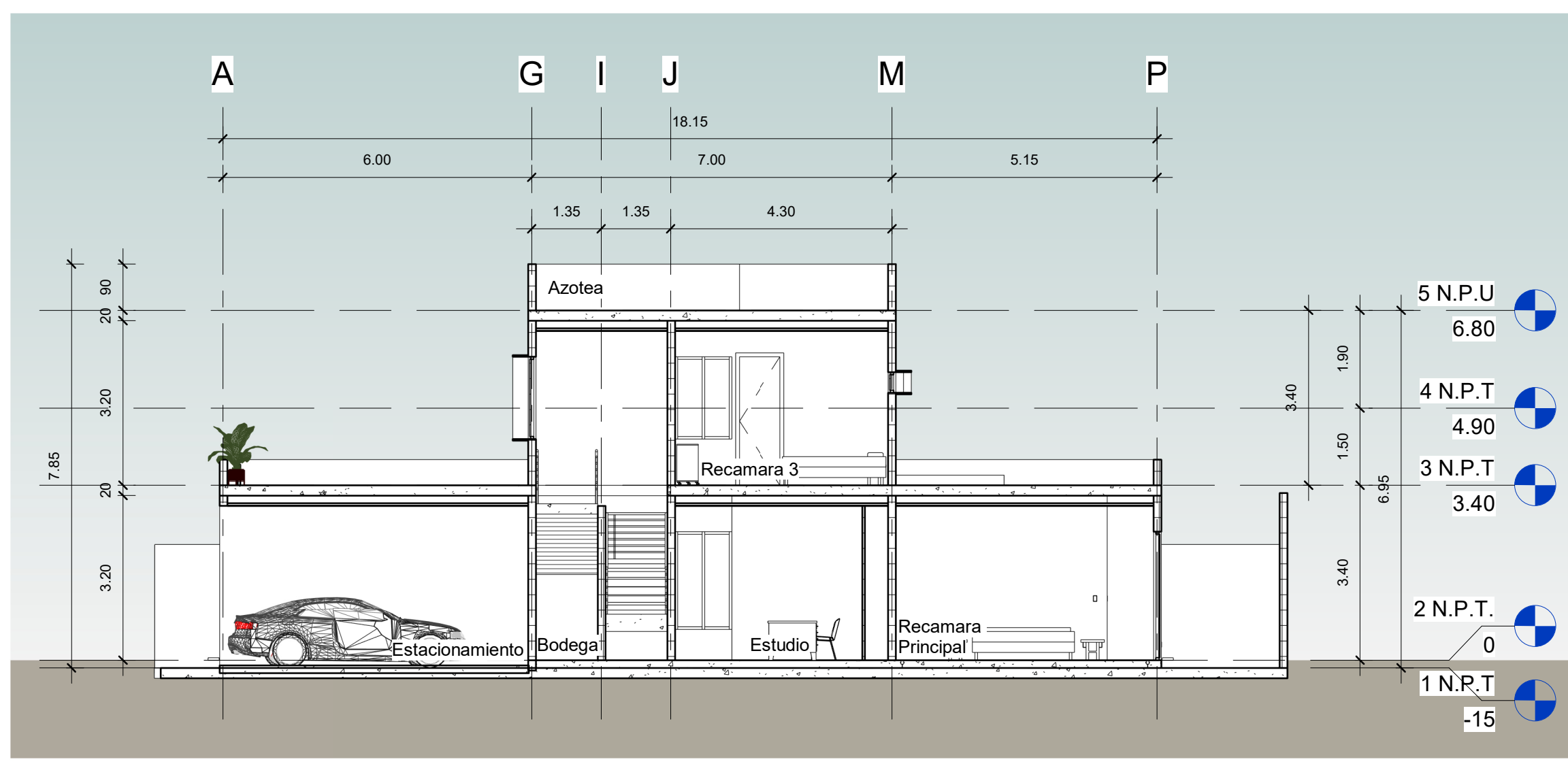
4 Sección 2 1 : 100
