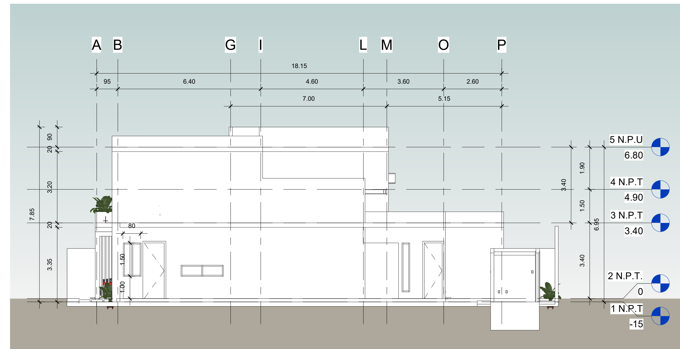
2 Fachada Sur 1 : 100
