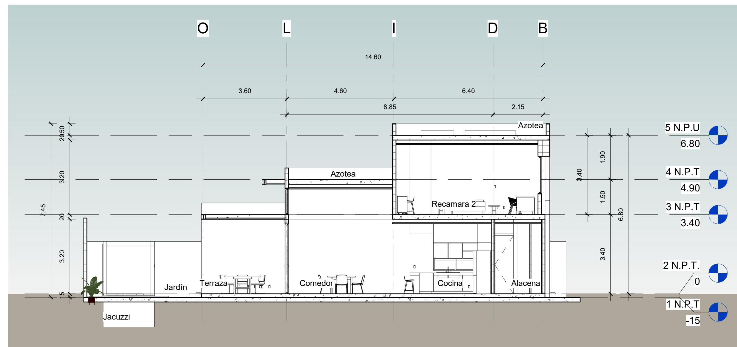
3 Sección 1 1 : 100
