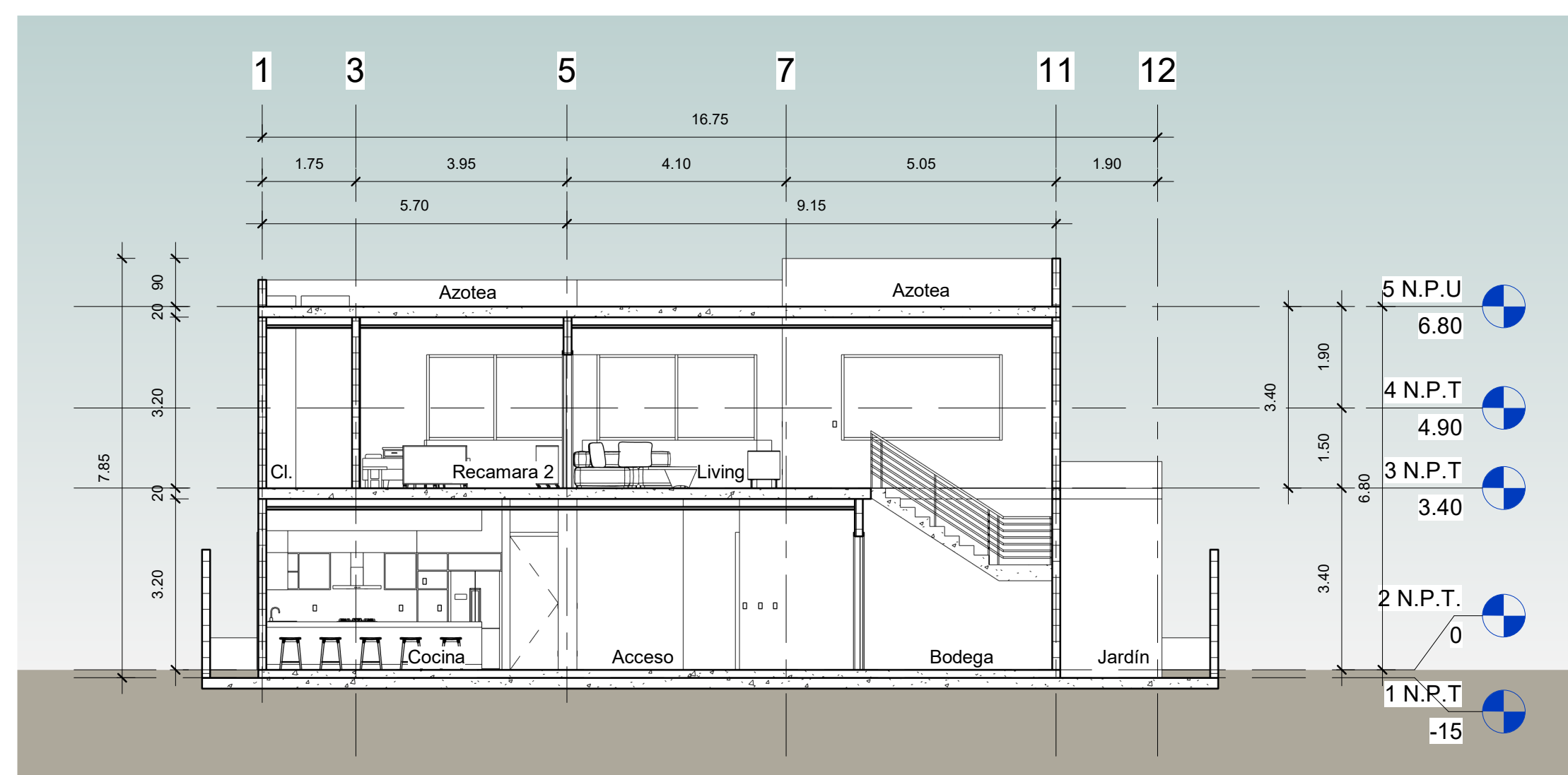
5 Sección 3 1 : 100
