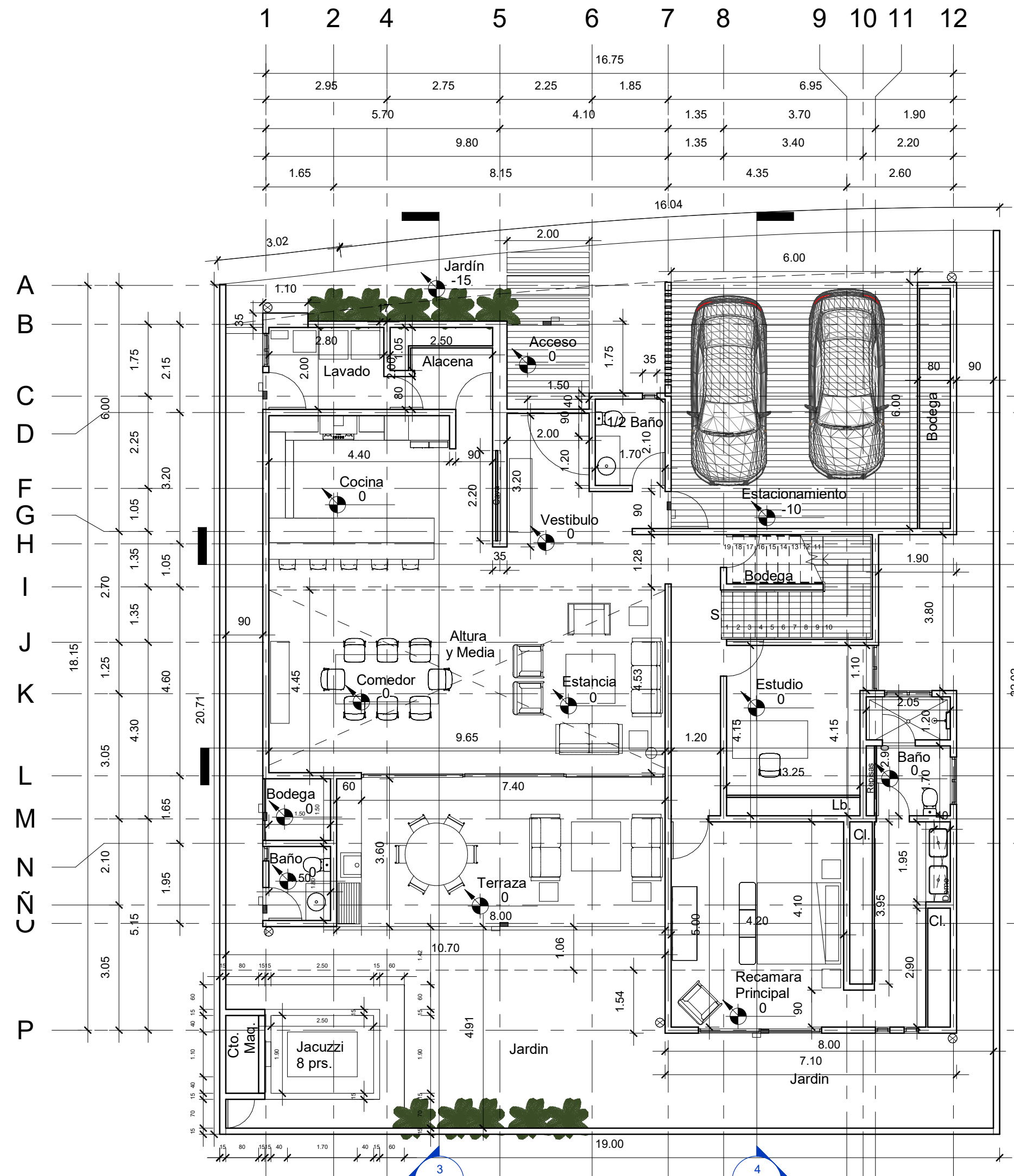
1 Planta Baja 1 : 100
