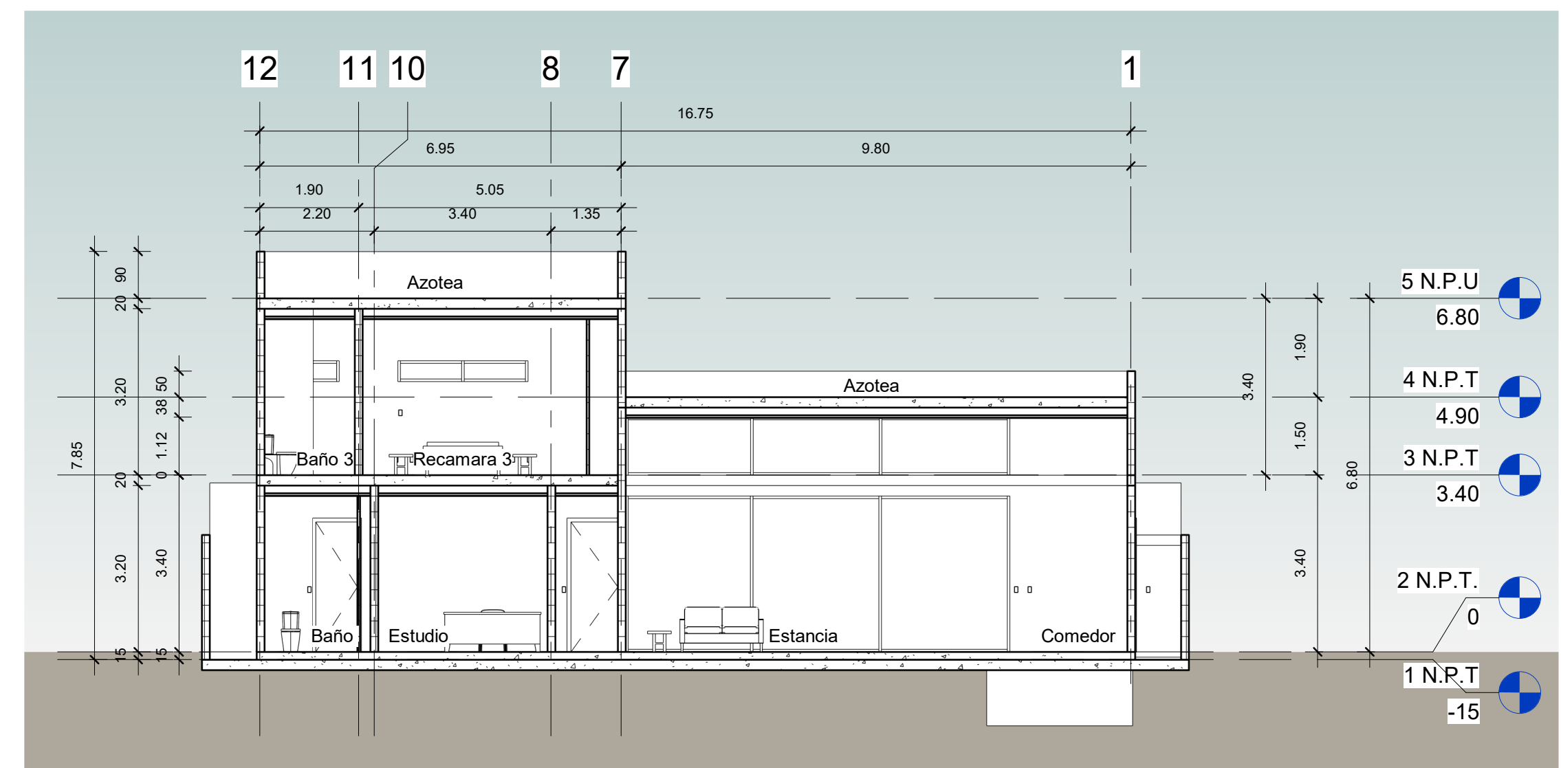
6 Sección 4 1 : 100
