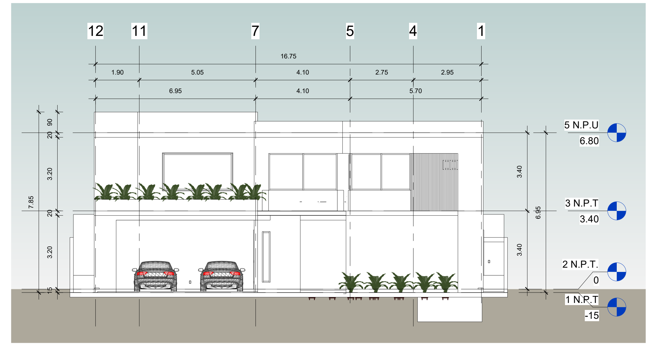
5 Fachada Oeste 1 : 100
