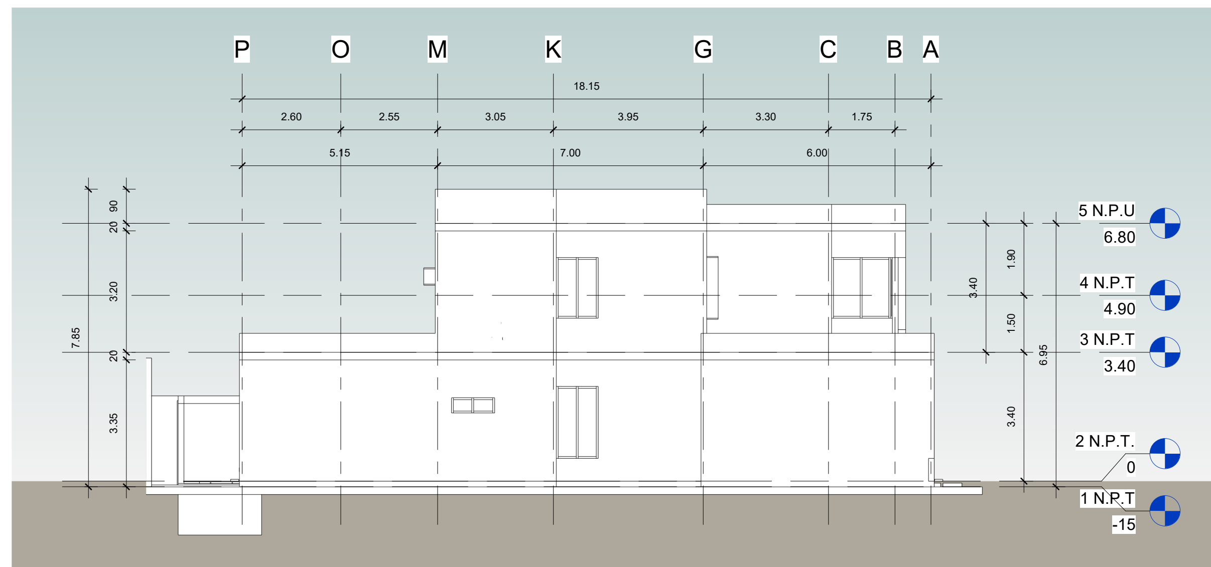
1 Fachada Norte 1 : 100
