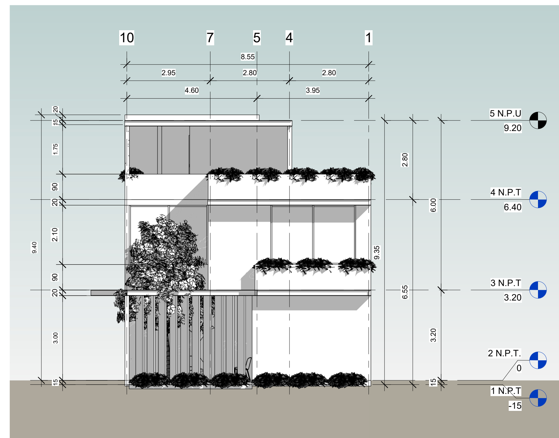
5 Fachada Norte 1: 75
