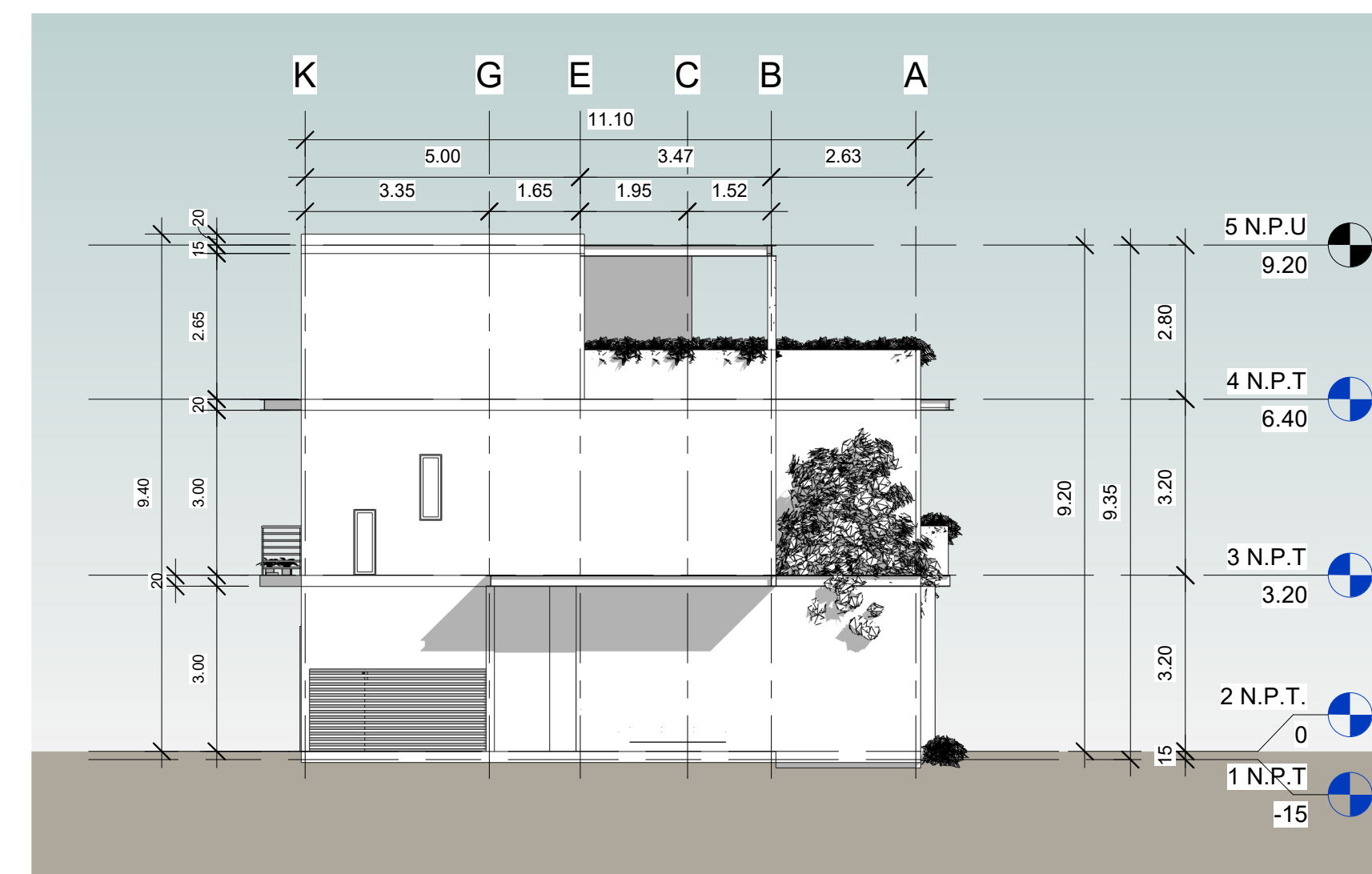
.1 Fachada Este 1: 100
