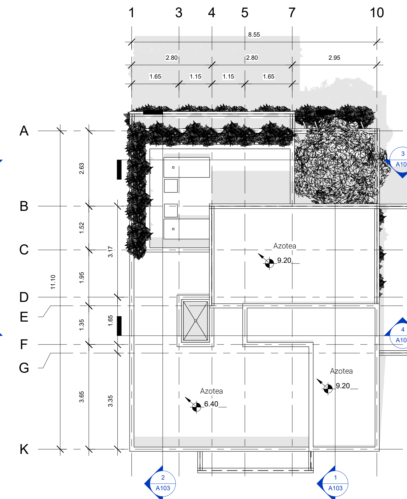
4 Planta Conjunto 1: 75
