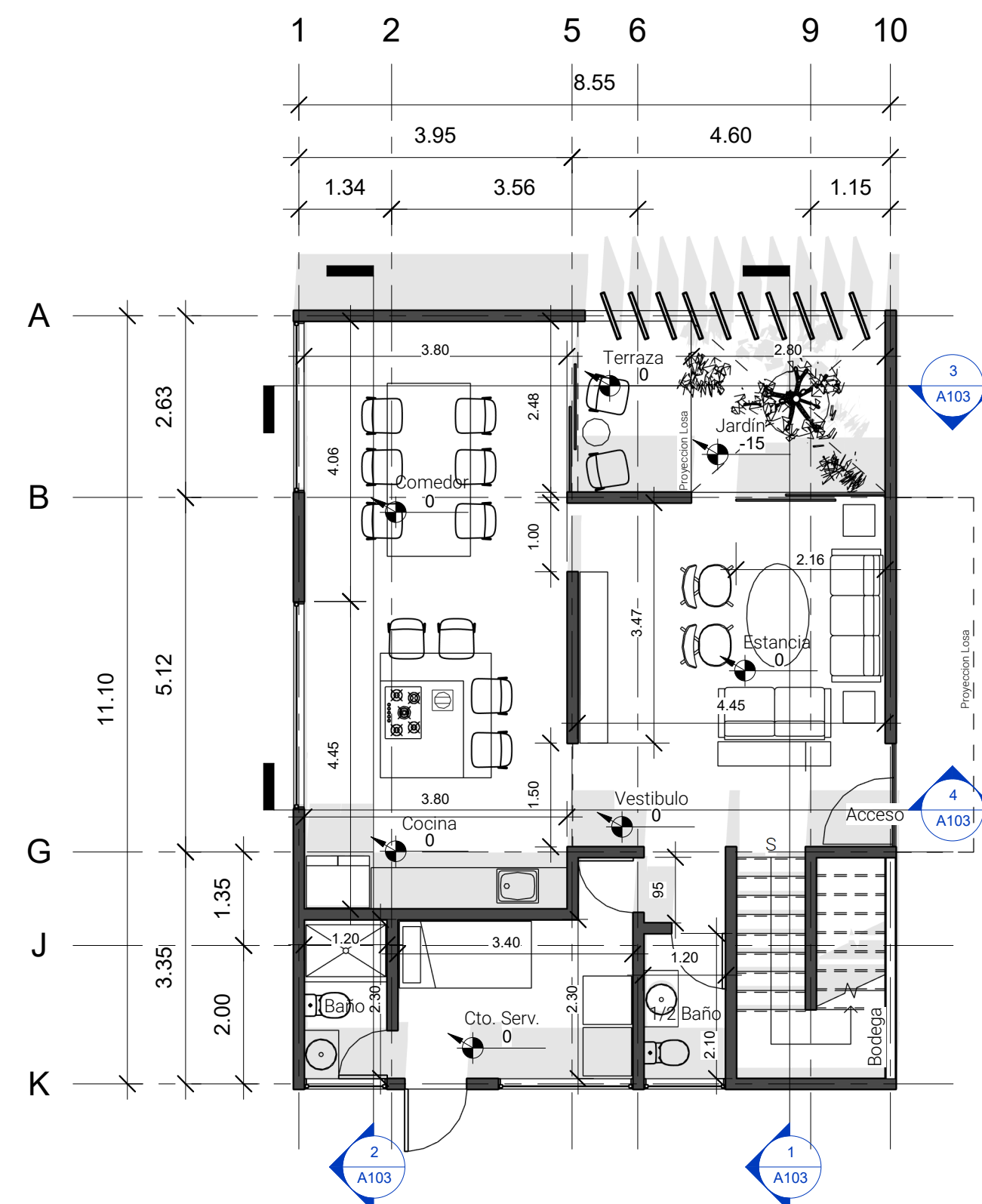
1 Planta Baja 1: 75
